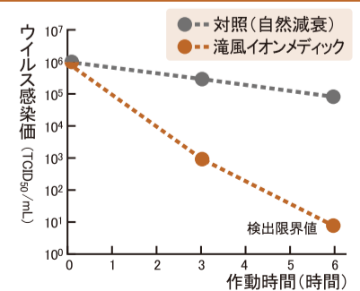
時間経過による付着ウイルス感染価の変化
