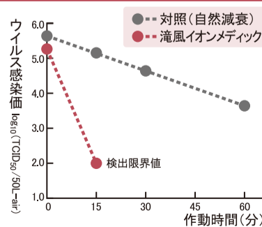
経過時間ごとの浮遊ウイルス感染価(対数値)の変化
